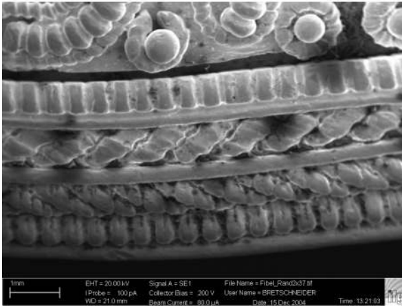
Abb. 4 Goldschmuck von Hiddensee, Detail der scheibenförmigen Fibel. Ornament (oben) und Randdekor (unten) aus Drähten mit unterschiedlicher Stärke und Struktur. Aufnahmen im Rasterelektronenmikroskop mit 37facher Vergrößerung.
